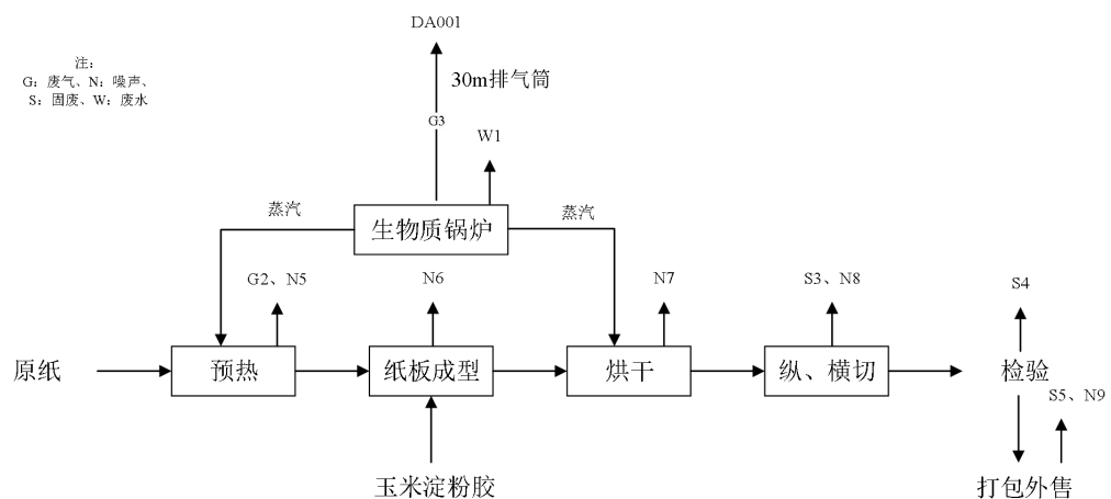
图 2-3 瓦楞纸板生产工艺流程图
