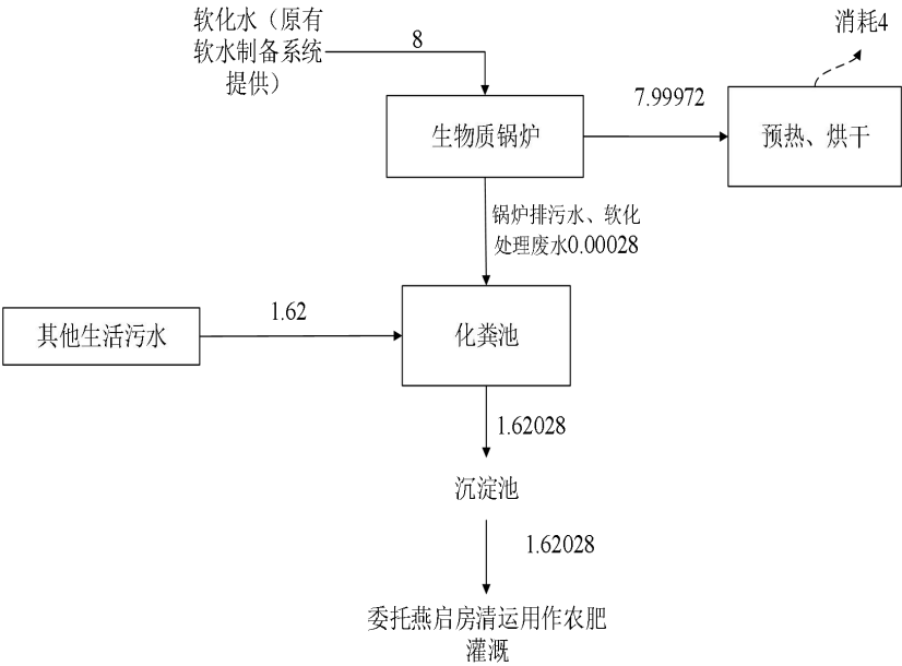
图 4-1 拟建项目水量平衡图 单位：m³/d
