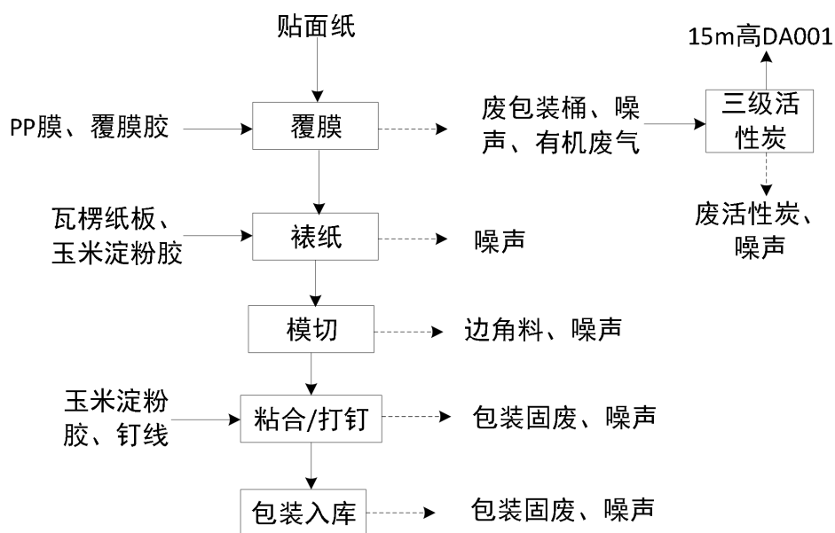
图 2-4 彩箱生产工艺流程图
