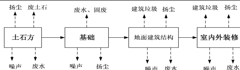
图 2-2 项目施工期工艺流程图
