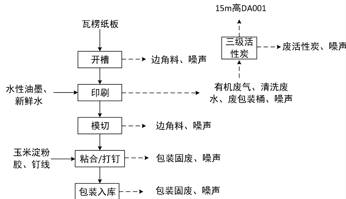
图 2-3 普通纸箱生产工艺流程图
