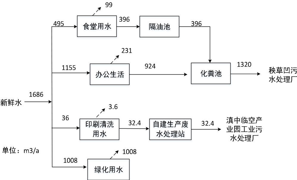
图 2-1 项目水量平衡图 (m³/a)
