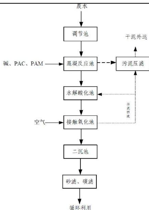
图 4-1 废水处理工艺流程图
