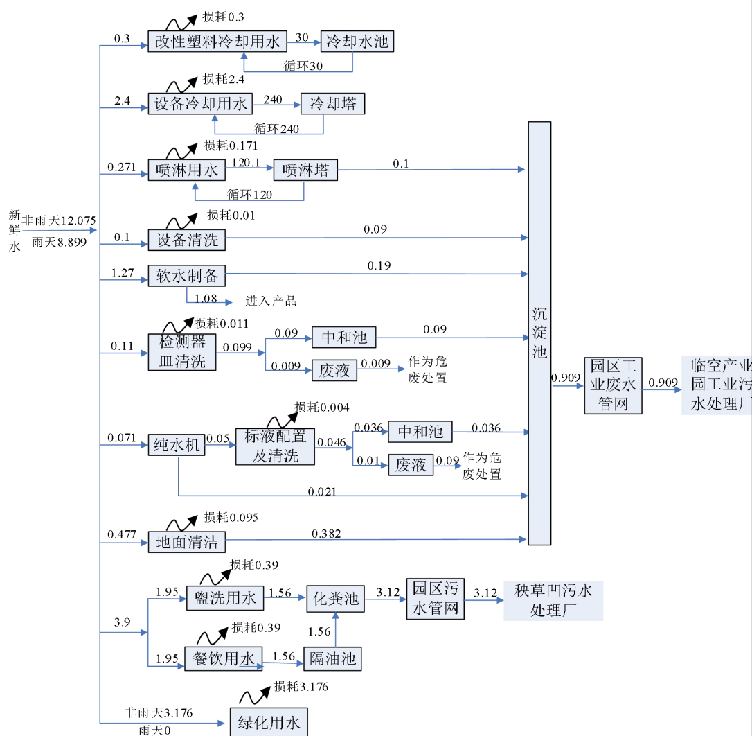
图 2-1 项目水量平衡图（单位：m³/d）
