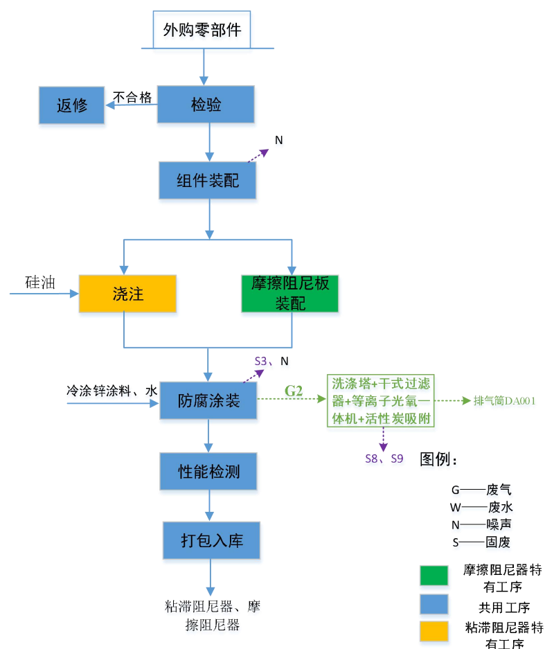
图 2-4 减震阻尼器生产工艺流程及产污环节图
