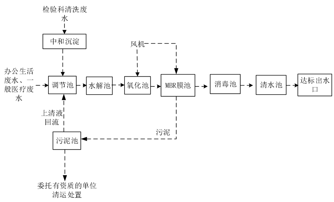
图4-1 污水处理站工艺流程图
