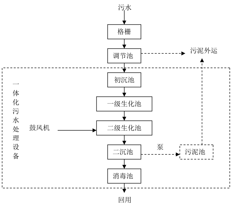
图 4-2 云南省第七强制隔离戒毒所化污水污水处理工艺
