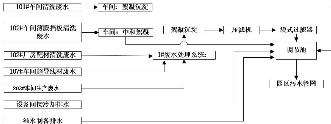
图 4-1 1#废水处理系统处理工艺流程图
