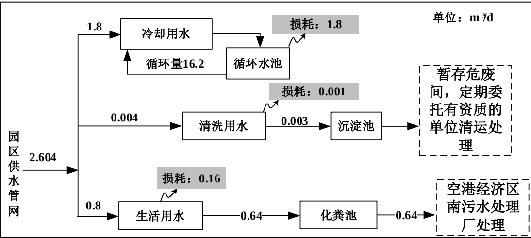
图 2-1 项目日水量平衡图
