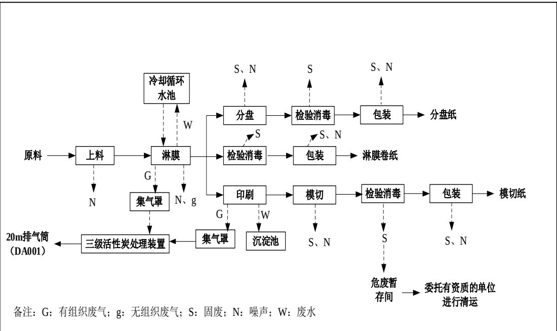
图 2-4 项目工艺流程及产污节点
