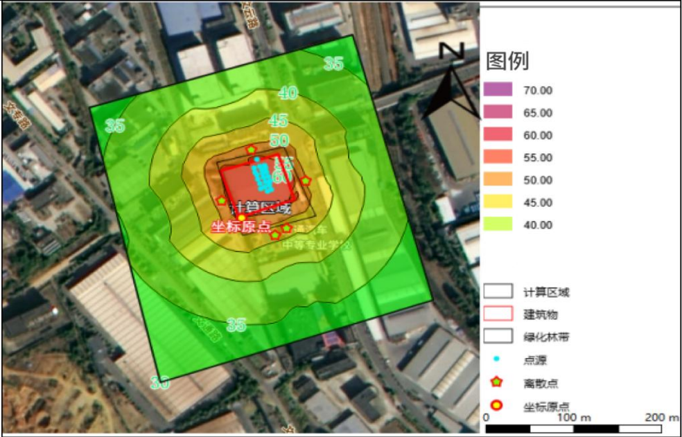
图 4-1 项目噪声预测等声值线图
