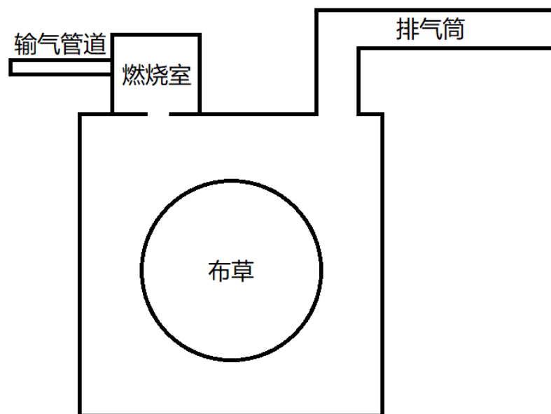
图 4-1 烘干机废气排放示意图
