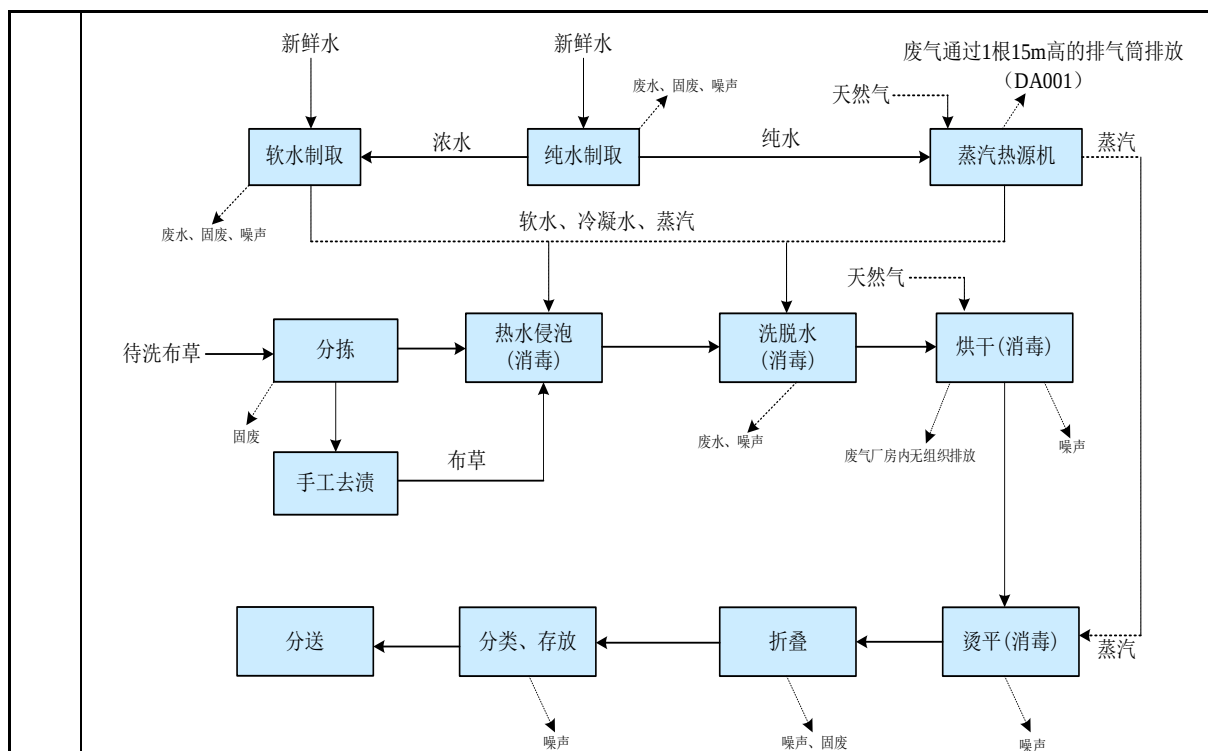
图 2-4 项目生产工艺流程及产污节点图
