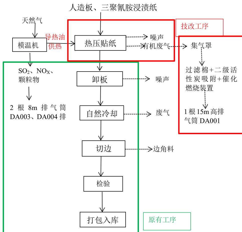
图2-4 饰面板工艺流程及产污节点图
