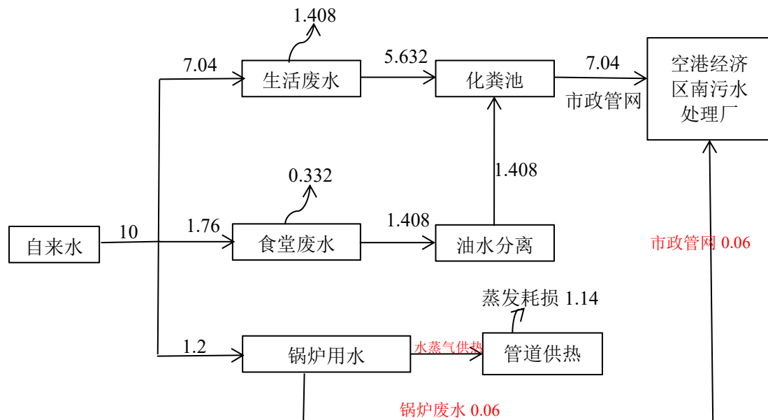
图 2-1 技改项目水量平衡图 单位 m³/d
