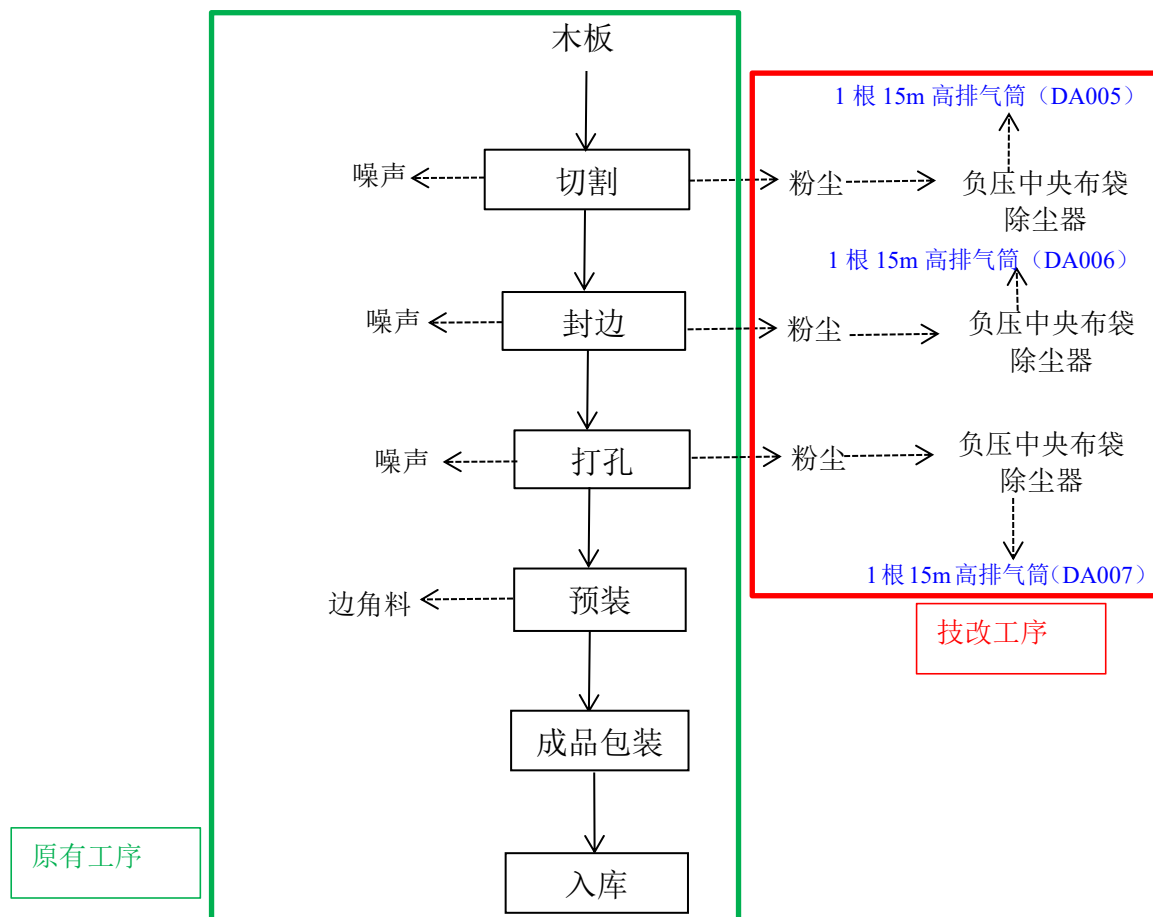
图 2-5 板式家具工艺流程及产污节点图
