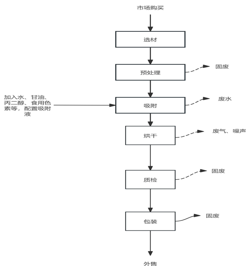
图 2-4 项目生产工艺流程及产污环节示意图（吸收法）
