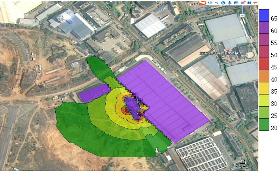
图 4-1 昼间贡献值等声级线图
